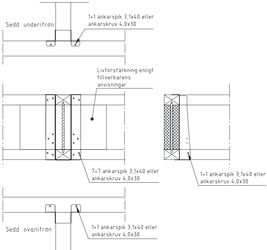
Figur 5. Montering av balksko typ H, alternativ B.
