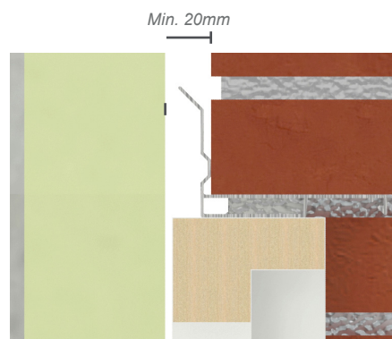
Muröppningsformens rygg är 20 mm djup, erforderligt utrymme måste därför finnas, till exempel genom en luftspalt eller inskärning i isolering.
