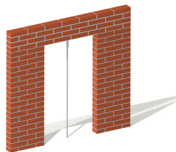
Stämpa muröppningsformen med cirka 1 m avstånd.
