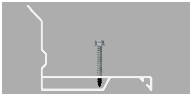
Tvärsnitt i längdriktningen som visar skruvarnas förankringsdjup.
