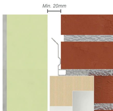
Muröppningsformens rygg är 20 mm djup, erforderligt utrymme måste därför finnas, till exempel genom en luftspalt eller inskärning i isolering.
