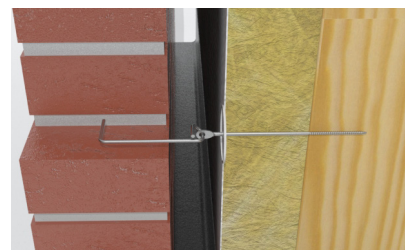
Montage av kramla i murverkets liggfog.
