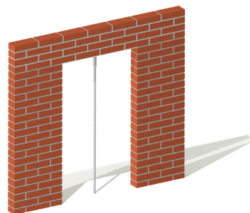
Stämpla muröppningsformen med cirka 1 m avstånd.
