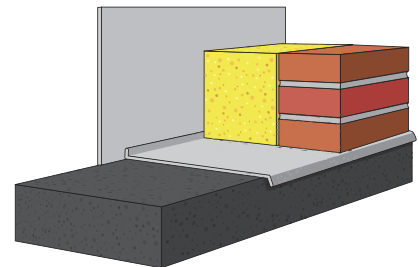
Princip för uppbyggnad av vägg med Jomas Grundplåt som glidskikt.
